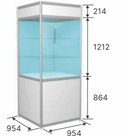
Spinta-vitrina su stiklais Show-case
