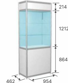
Spinta-vitrina su stiklais Show-case
