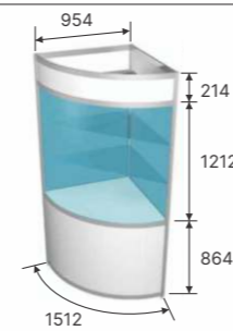
Kampinė vitrina (lenkta) Corner show-case (arched)
