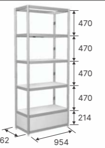
Lentynų konstrukcija Shelves construction
