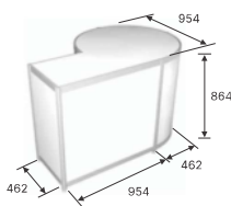
Stalas - baras Bar table
