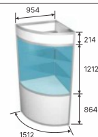
Kampinė vitrina (lenkta) Corner show-case (arched)
