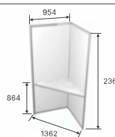
Kampinė lentyna Corner shelf
